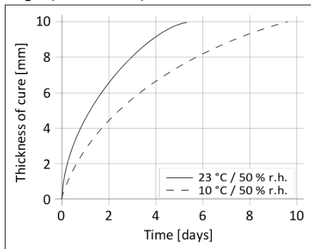
Schema 1: Uithardingsnelheid voor Sikaflex®-298 FC
