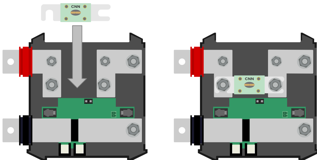
Het plaatsen van de CNN-zekering in de Lynx Shunt VE.Can
