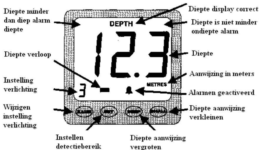
FIGUUR 3 - Het standaard display
