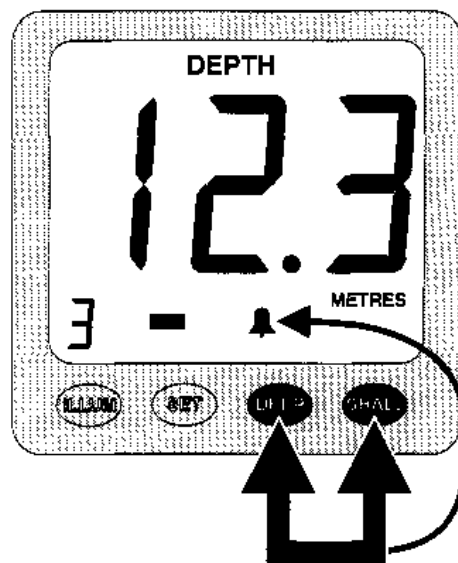
FIGUUR 7 - Activeren en uitschakelen van de alarmen
