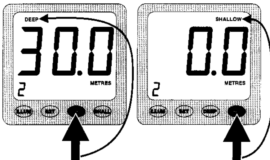
FIGUUR 6 - Selectie van het diepte of ondiepte alarm
