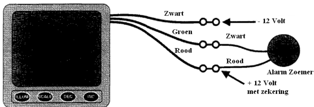
FIGUUR 1 - Elektrische Aansluitingen
